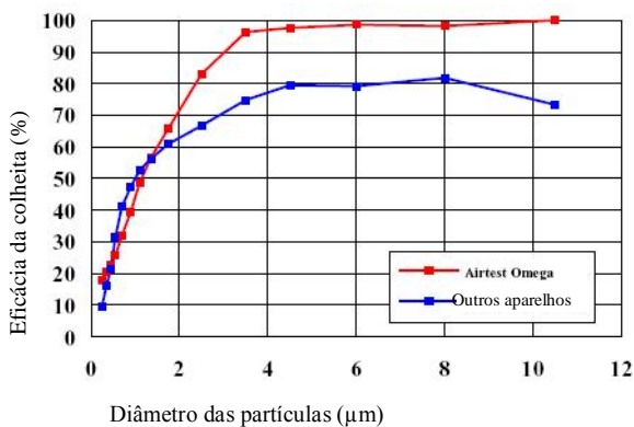
Curva de eficácia da colheita do AIRTEST OMEGA
